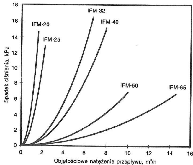
Rys. nr 4. Charakterystyka hydrauliczna filtrów IFM
